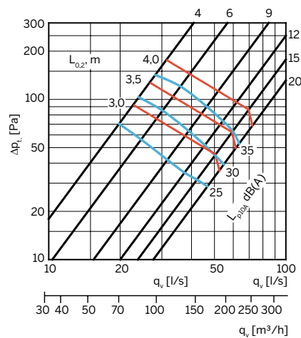
TVZ 160
