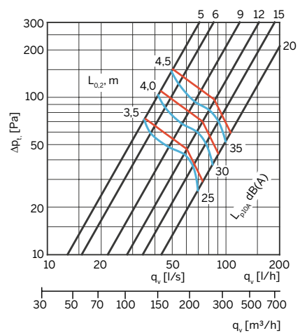
TVZ 200
