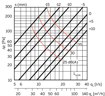
TVLNA-M-SD 100
