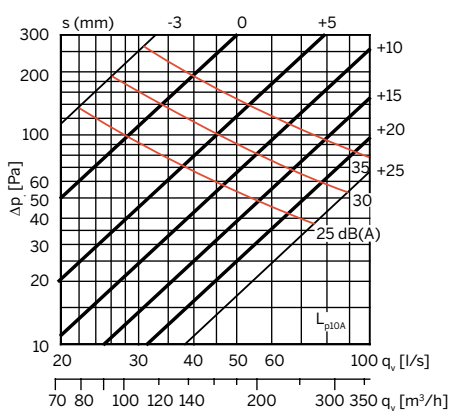
TVLNA-M-SD 200
