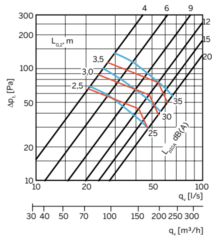
TVZ 150
