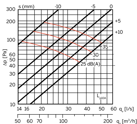
TVLNA-M-SD 125
